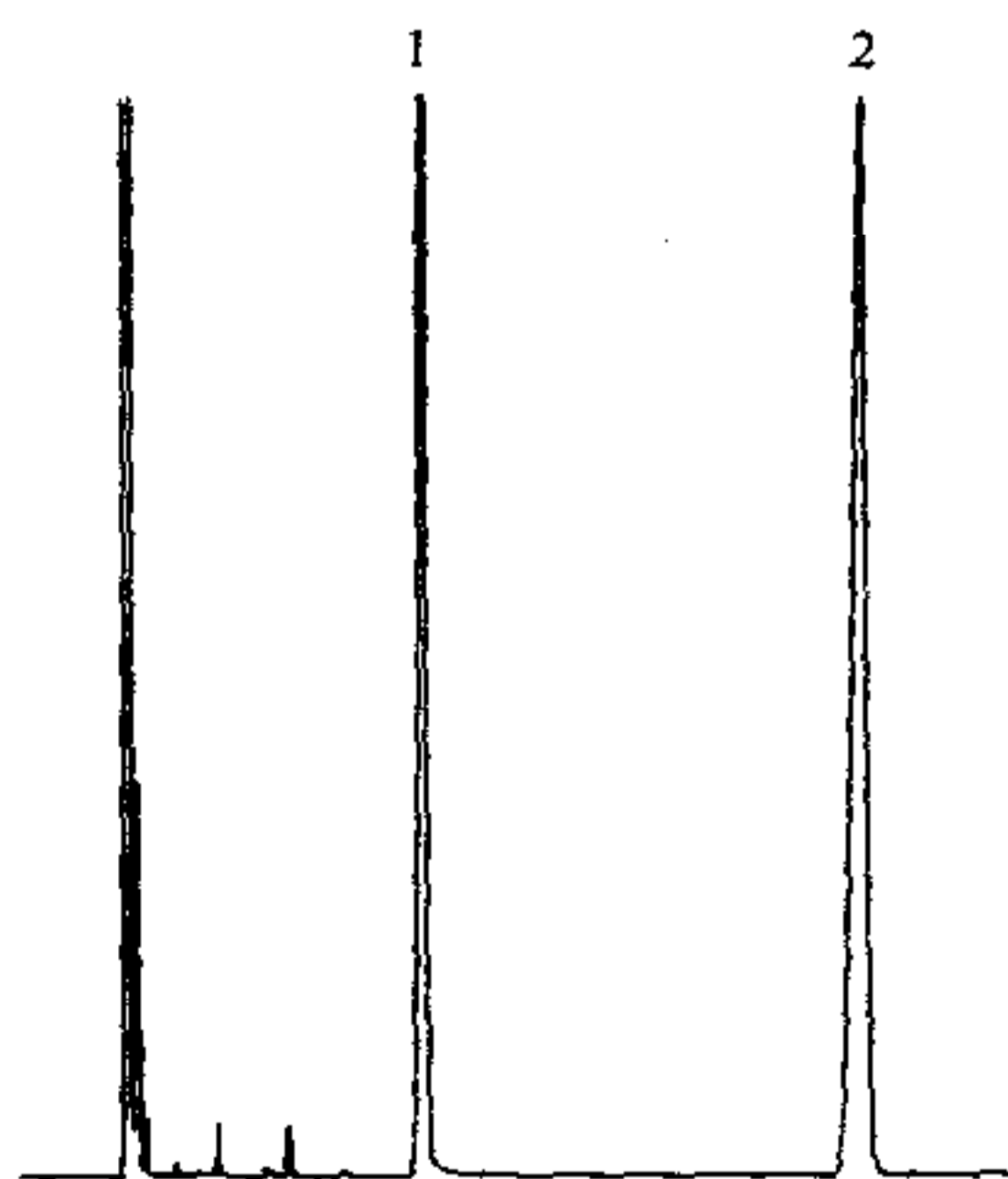
图 A.1 稻瘟灵乳油毛细管气相色谱图
