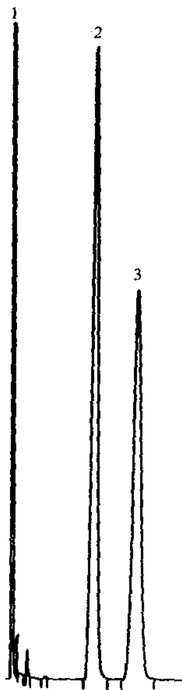
1—溶剂；2—稻瘟灵；3—内标物(正二十二烷)
